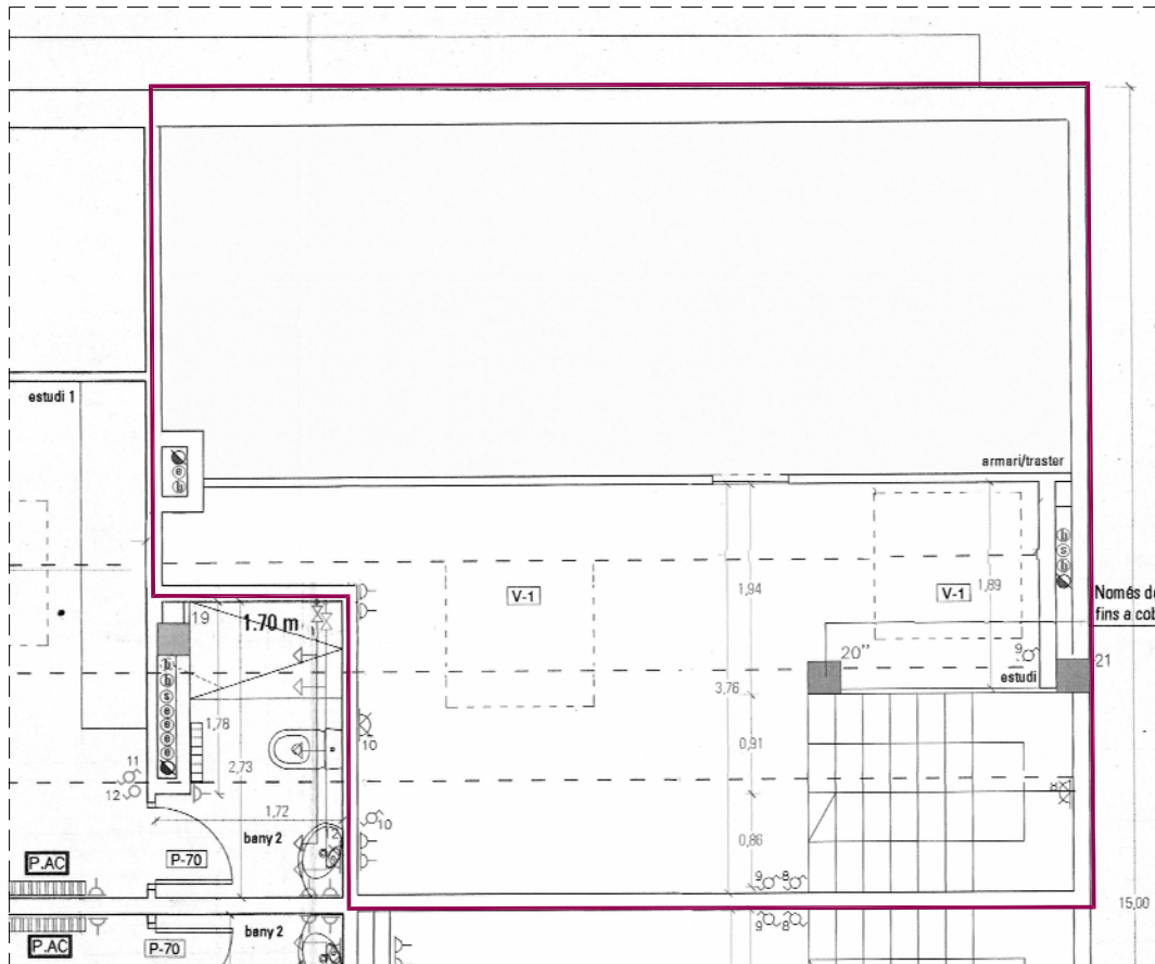
PLANTA SOTACOBERTA
